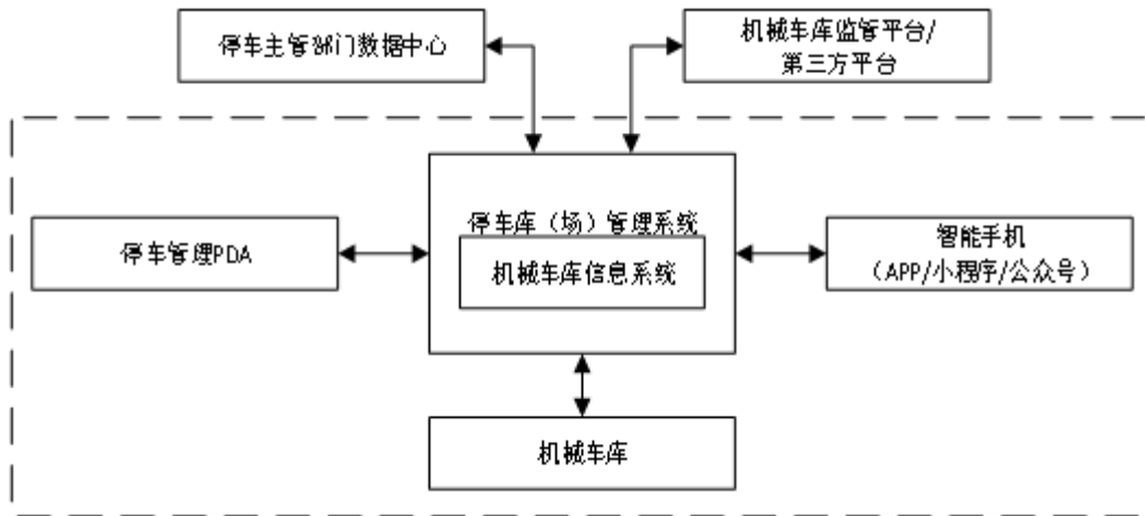
图1 场内机械车库信息系统
